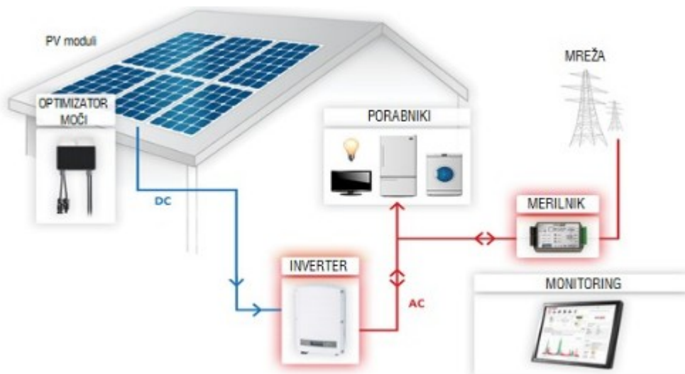
Slika 2: Shematski prikaz osnovnih komponent sončne elektrarne za lastno rabo
