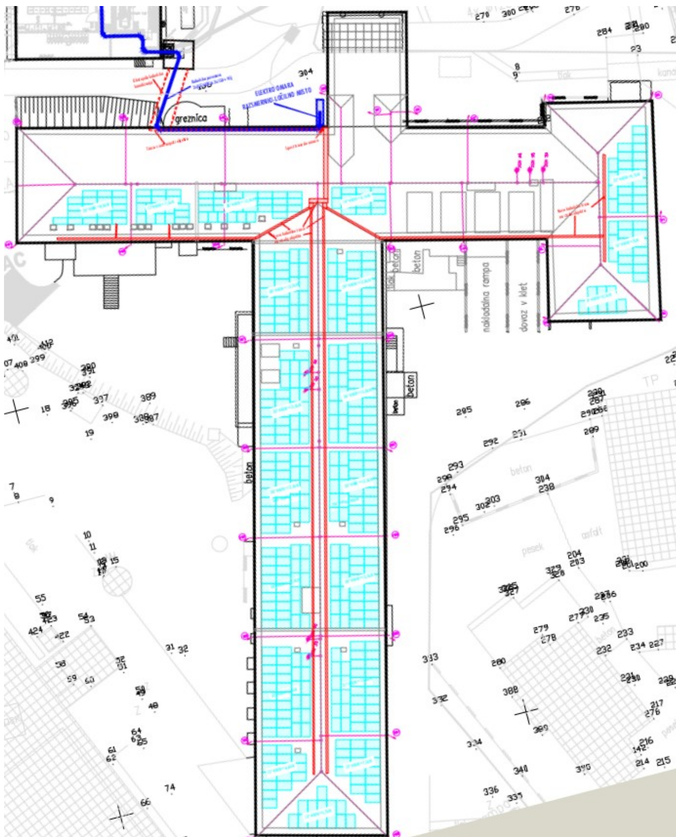
Slika 4: Tloris strehe objekta kjer bo nameščena sončna elektrarna
